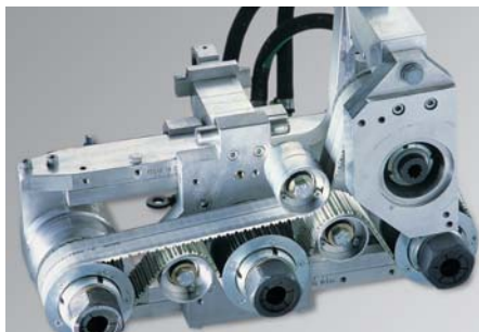
Trapano idraulico a tre teste
