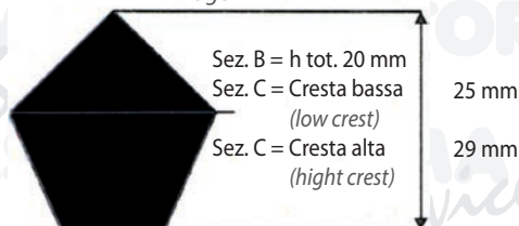
Crestatura Ridge
