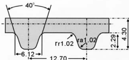
Profilo H
