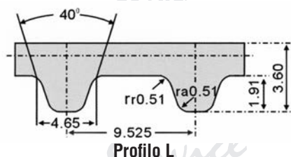
Profilo L
